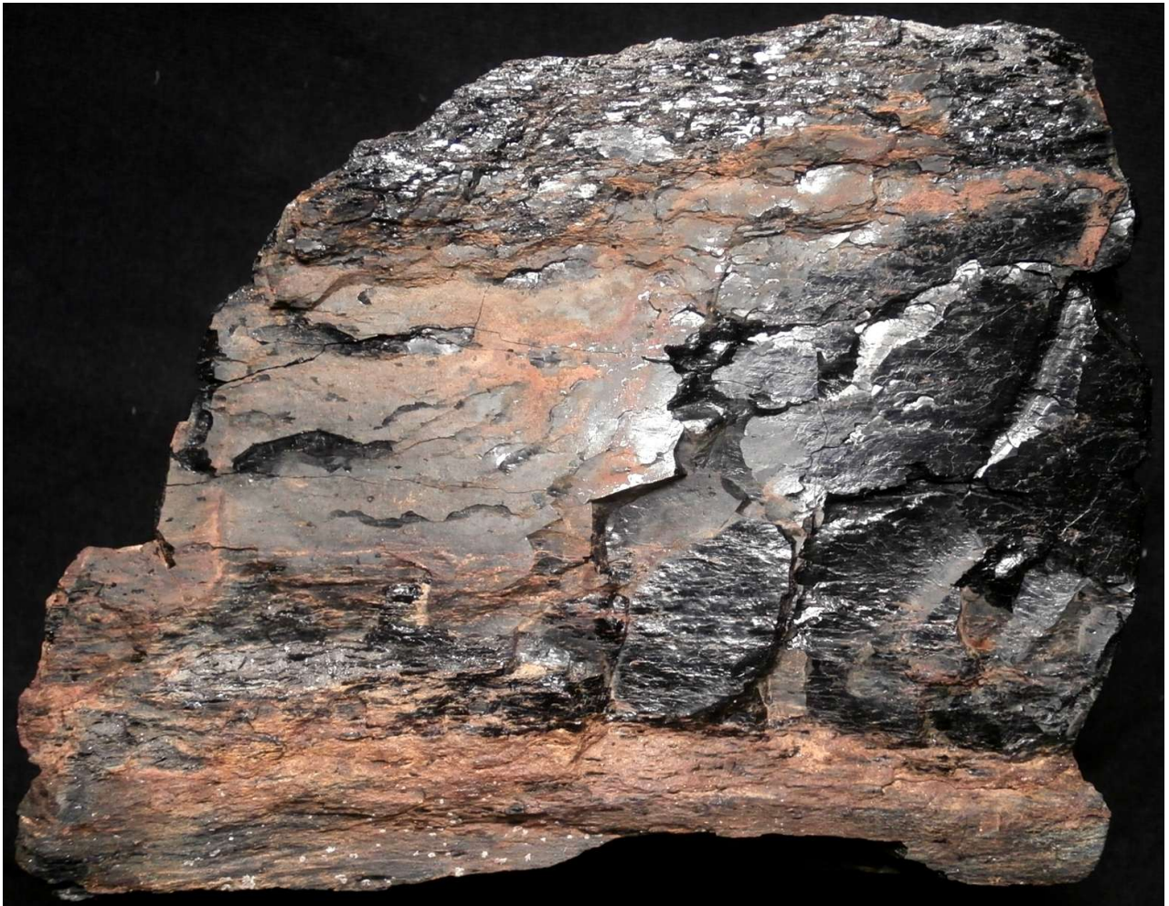
Angewitterte Kohle aus dem Anstehenden im Stammeregg-Bach. Die etwa 9 cm hohe Probe repräsentiert die gesamte Dicke des Flözchens. Fund 2.11.2025, Nr. 5605, Breite des Stücks ca. 11.5 cm.
